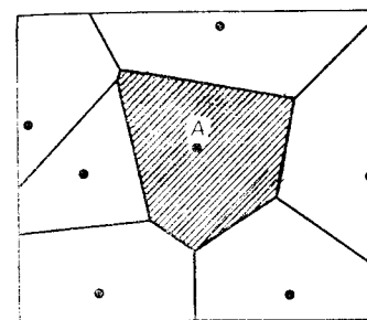
Рис. 5.45. Многоугольник Тиссена (заштрихован) вокруг точки A.
