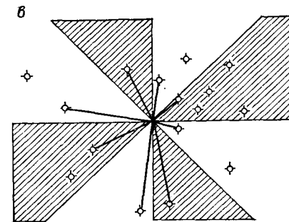
Рис. 5.57. (а) Метод поиска, локализирующий n ближайших соседей вокруг оцениваемого узла сети. На радиальное распределение контрольных точек не накладывается никаких ограничений. (б) Схема поиска по квадратам, используемая для установления истинного распределения контрольных точек вокруг оцениваемых узлов сети. (в) Октантный вариант схемы поиска вокруг оцениваемых узлов сети
