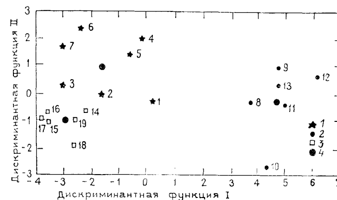
Рис. 6.51. Представление нагрузок на дискриминантные функции I и II: 1 — доломиты Элленбургера; 2 — доломиты Грейбурга; 3 — известняк Виола; 4 — центры групп. 1—19 — номера проб
