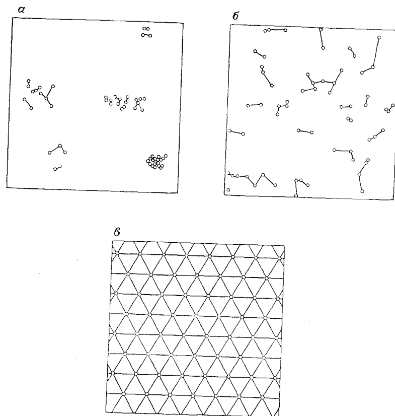
Рис. 5.14. Значения статистик метода ближайшего соседа R для различных схем расположения точек на картах (по Р. А. Ома, 1984): a — точки сгруппированы в пять групп, R=0,34 ; b — точки рассеяны случайно, R=0,91 ; c — точки размещены по шестиугольной сети, R=2,15 . Плотность точек \lambda одинакова для всех схем
