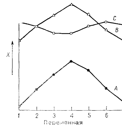
Рис. 6.9. Графики переменных, измеренных на трех объектах.
