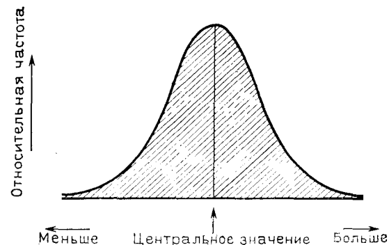
Рис. 2.9. График плотности нормального распределения
