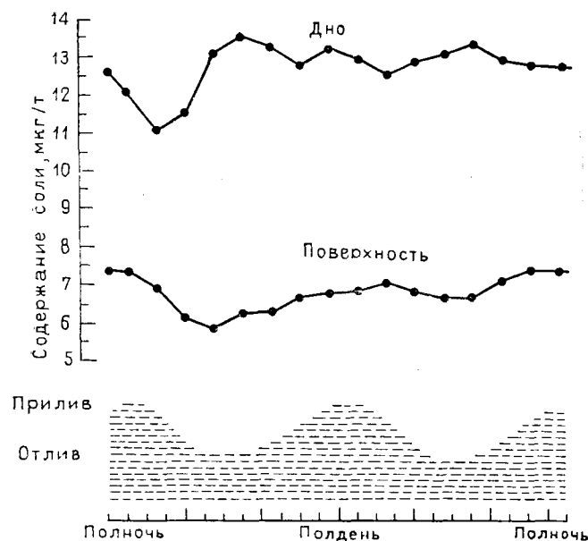
Рис. 4.38. Содержания соли в придонных водах и поверхностных водах и Шизапик Бей вблизи Аннаполиса (штат Мэриленд)
