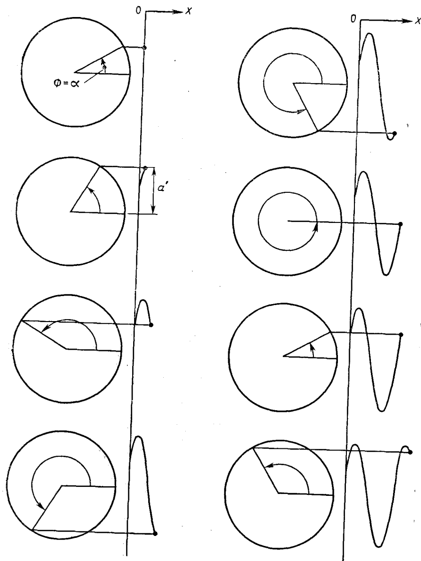
Рис. 4.51. Постепенное изменение фазового угла от начального значения \Phi . Для последовательных значений x , Y_1 = A \sin(2\pi x_1/X + \Phi) и a_1 = 2\pi x_1/X + \Phi
