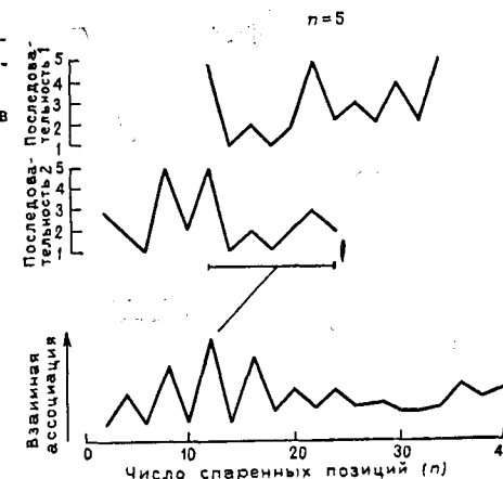
Рис. 4.40. Сравнение двух нечисловых последовательностей с помощью метода взаимосвязей. Две последовательности изображены в положении максимума сходства
