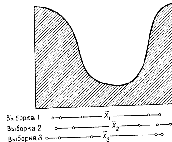
Рис. 2.24. Три выборки из пяти наблюдений, взятые наудачу из совокупности с U-образным распределением. Средние значения выборок обозначены черз \bar{X}
