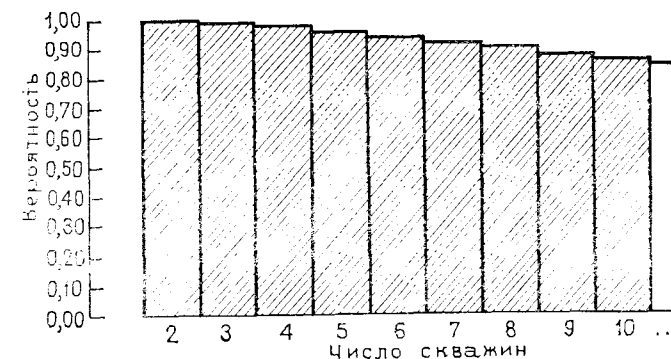
Рис. 2.5. Дискретное распределение, дающее вероятность того, что будет пробурено больше заданного числа скважин, для того, чтобы получить два успеха, при условии, что вероятность успеха равна 10%
