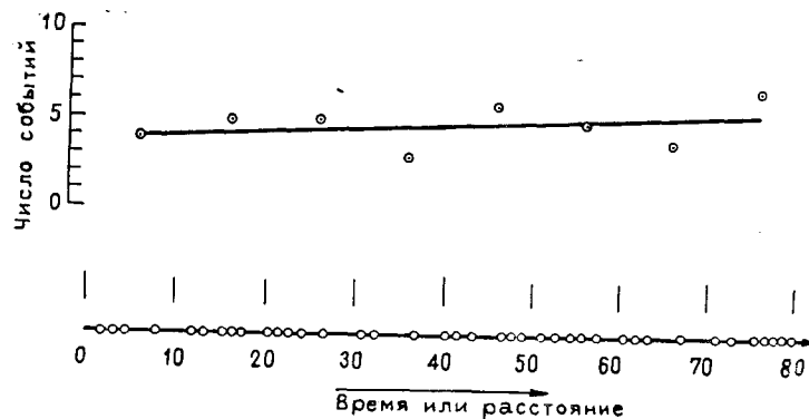
Рис. 4.10. Последовательности событий, которые происходят «мгновенно» в пространственном или временном континууме.
