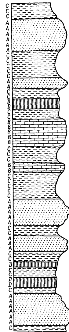
Рис. 4.4. Стратиграфический разрез, в котором литологические состояния взаимно исключают друг друга:
