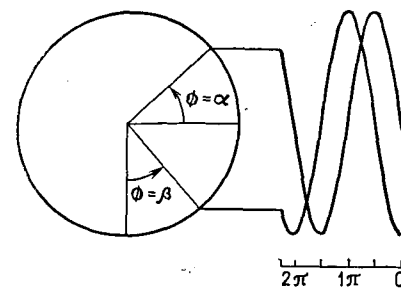
Рис. 4.52. Синусоидальная и косинусоидальная волны, соответствующие вращению диска.
