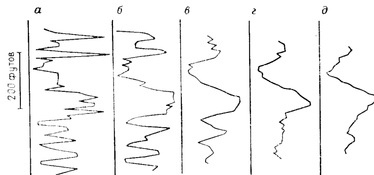
Рис. 4.60. Результаты сглаживания последовательности значений каротажной диаграммы в скважине с помощью различных уравнений [26, рис. 4.2]:
