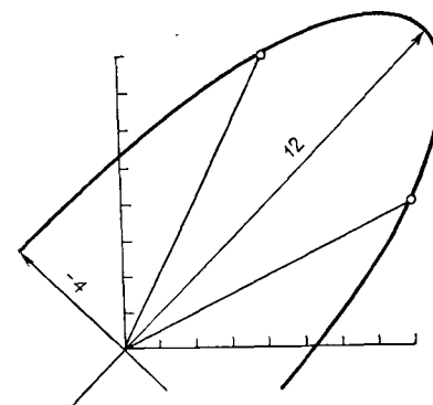
Рис. 3.2. Эллипс, определенный элементами матрицы порядка 2 \times 2 . Собственные векторы матрицы соответствуют главным полуосям эллипса
