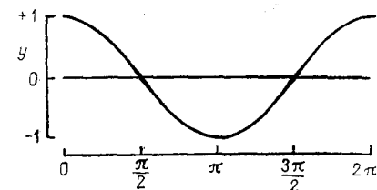
Рис. 4.53. Синусоидальная волна. Общая длина кривой равна 2\pi радиан
