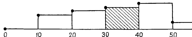
Рис. 4.3. Равномерная пространственная последовательность, полученная из неравномерно расположенных данных путем прямоугольного интегрирования. Площадь заштрихованной области такая же, как и на рис. 4.2
