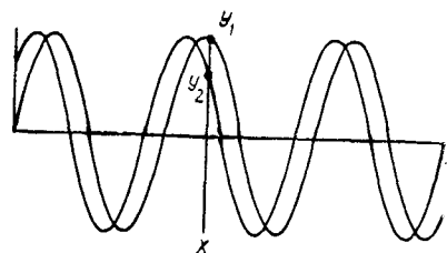
Рис. 4.49. Две синусоидальные волны, которые идентичны по форме. Различия между y_1 и y_2 для специфического значения x характеризуют разность фаз двух волновых форм
