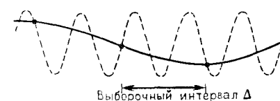
Рис. 4.57. Високонэнергетическая синусоидальная волна (прерывистая линия), наблюдаемая в дискретном множестве точек, дает отчетливо видную волну низкой частоты (сплошная линия)
