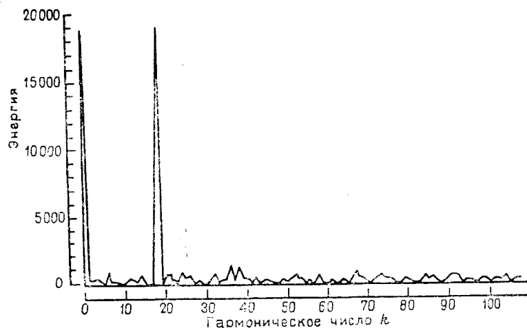
Рис. 4.55. Периодограмма месячного потока Кейв-Крик, Кентукки. Специальные значения указывают, что поток имеет единственный периодический годичный цикл. Энергии приведены в квадратах единиц измерения, которые равны сотням частей дюйма
