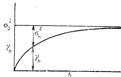
Рис. 4.43. Соотношение между полудисперсией \gamma_h и автоковариацией для стационарной регионализованной переменной. \sigma_0^2 — дисперсия наблюдений или автоковариация для лага 0. Для значений вне этого множества \gamma_h = \sigma_0^2
